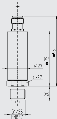
Salida de cable IP68 Prensaestopa no ajustables
