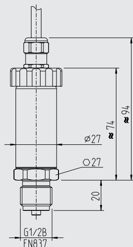
Salida de cable IP68 PUR (utilización permanente en el medio) no ajustables
