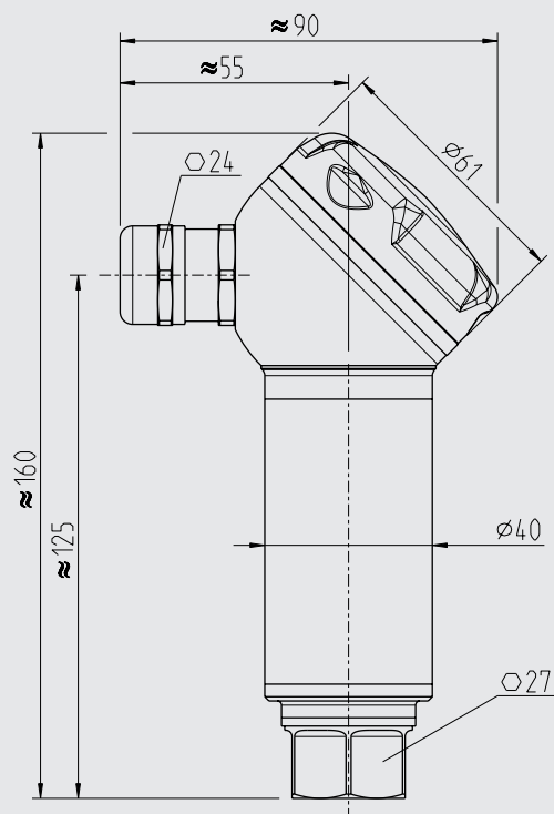
Caja de campo Prensaestopa ajustable
