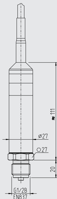
Salida de cable IP68 PUR (utilización permanente en el medio) no ajustables
