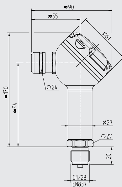
Caja de campo Prensaestopa ajustable
