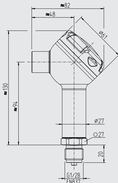
IS-3 para temperaturas del medio opcionales -40 ... +150 °C [-40 ... 302 °F] y -40 ... +200 °C [-40 ... +392 °F]
