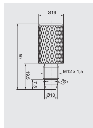
Espiga para soldar M12
