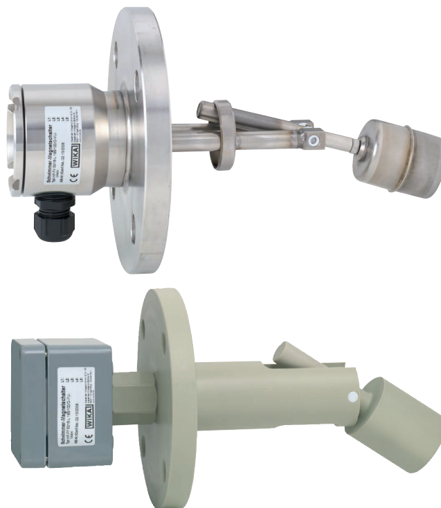
Fig. superior: versión en acero inoxidable, modelo HLS-S Fig. inferior: versión en plástico, modelo HLS-P
