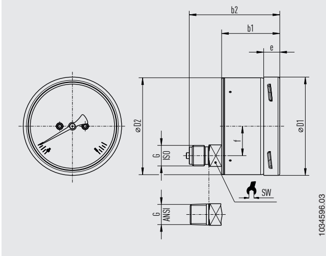
Modelo 232.30, conexión dorsal inferior
