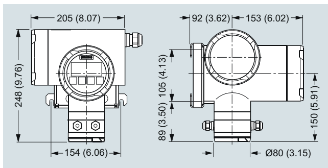
Transmisor SITRANS FM TRANSMAG 2 con soporte de montaje en pared especial, dimensiones en mm (inch)
