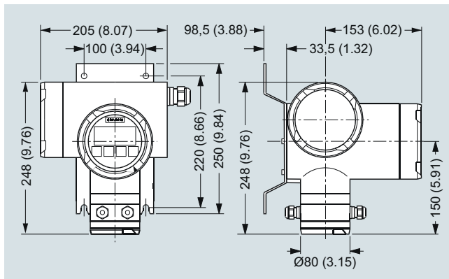
Transmisor SITRANS FM TRANSMAG 2 con soporte de montaje en pared, dimensiones en mm (inch)
