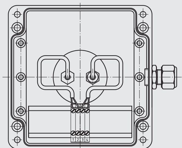
Borne de conexión
