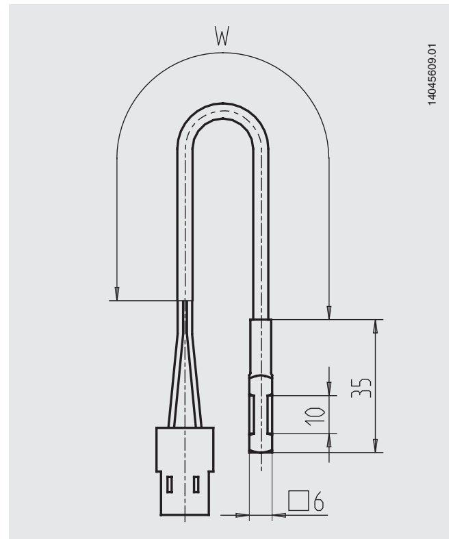
Modelo TF44 con conector
