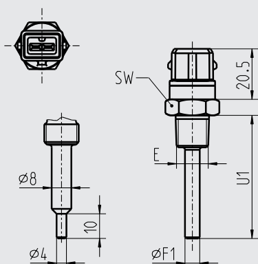
Conector de bayoneta, DIN 72585
