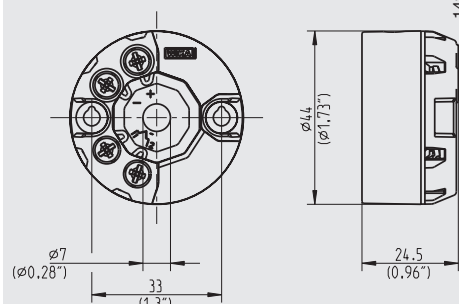
Versión de cabezal, modelo T16.H
