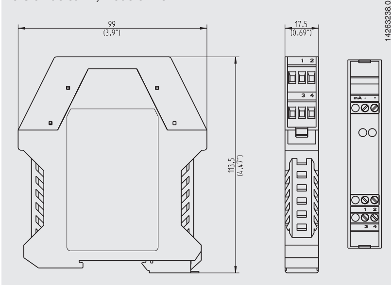
Versión de carril, modelo T15.R
