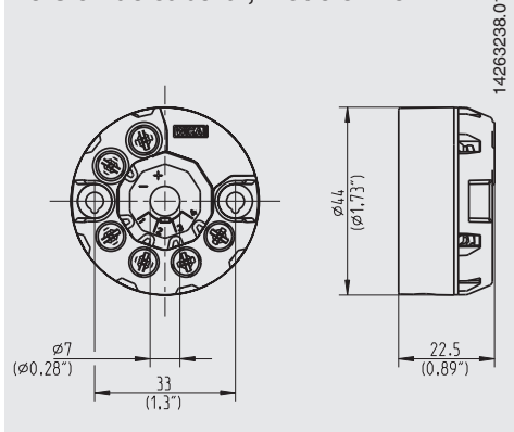
Versión de cabezal, modelo T15.H
