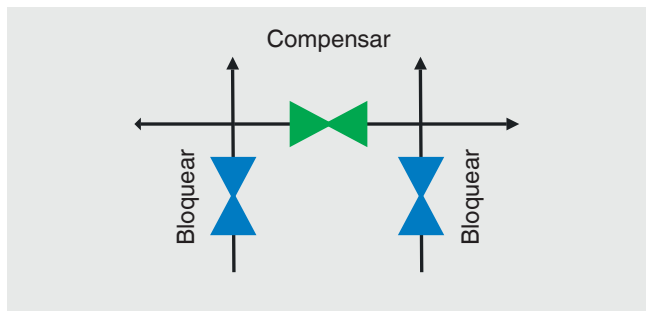
Manifold 3 válvulas
