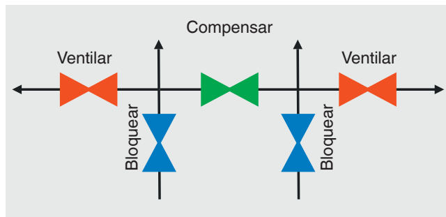
Manifold 5 válvulas
