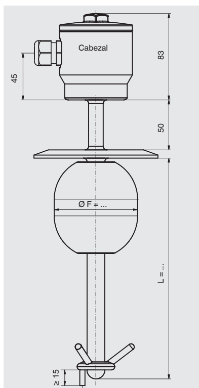
Con soporte de flotador separado
