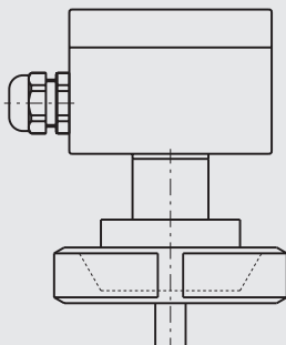
Racor roscado según DIN 11851
