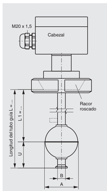
Racor roscado según DIN 11851
