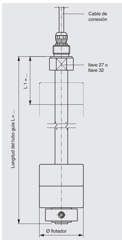
Versión con rosca y cable de conexión
